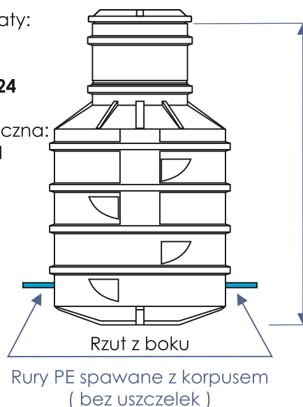
Studzienka wodomierzowa SW100
