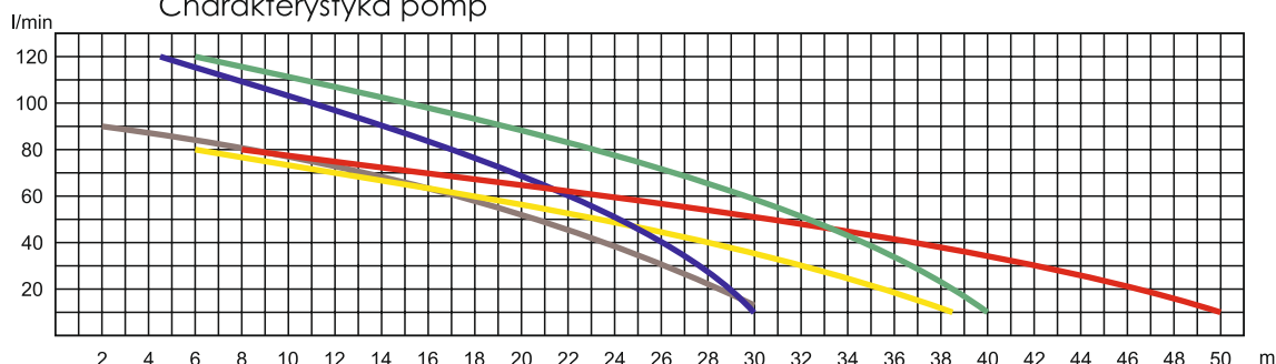
Charakterystyka pomp
