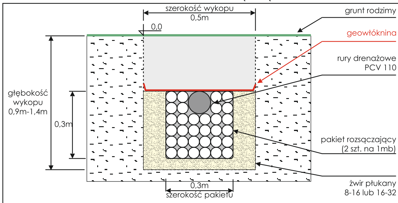
PRZEKRÓJ POPRZECZNY PRZYKŁADOWEGO PAKIETU ROZSACZAJĄCEGO PRO-1R DO DRENAŻU
